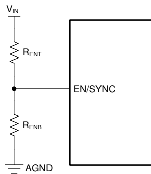
Figure 9. VIN UVLO Using the EN pin
